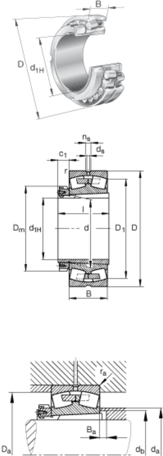
FAG 230/710-B-K-MB + H30/710图片
