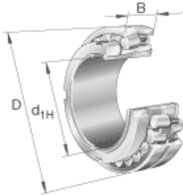
FAG 230/500-B-K-MB + H30/500图片
