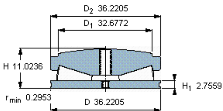
球面垫圈的半径 R 2300
