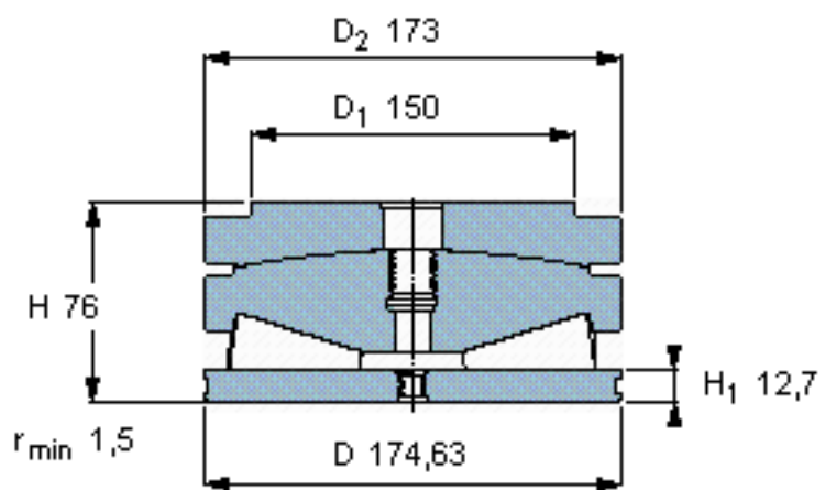
球面垫圈的半径 R 457,2
