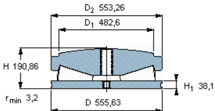
球面垫圈的半径 R 1270
